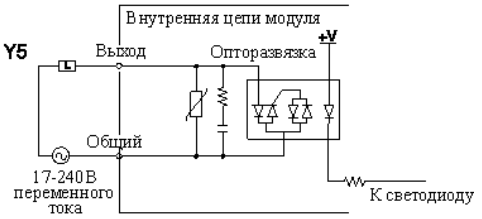
Эквивалентная схема выхода
