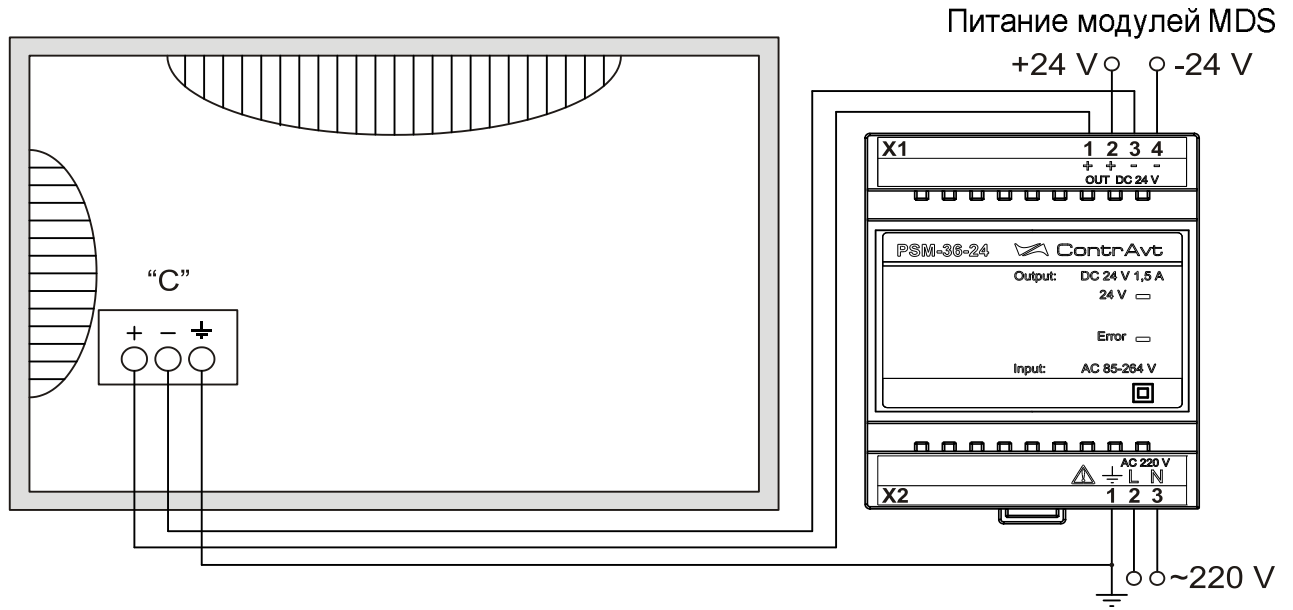
Рисунок 5 – Подключение электропитания
