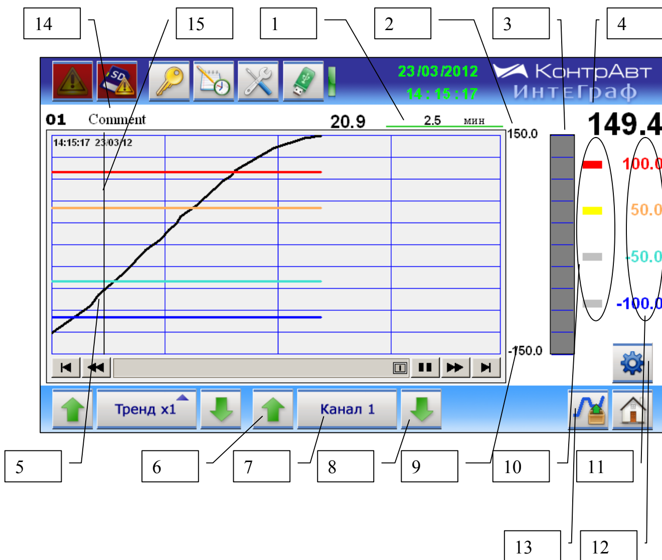
Рисунок 8 – Внешний вид экрана Единого тренда аналогового измеренного сигнала ( Тренд x1 )
