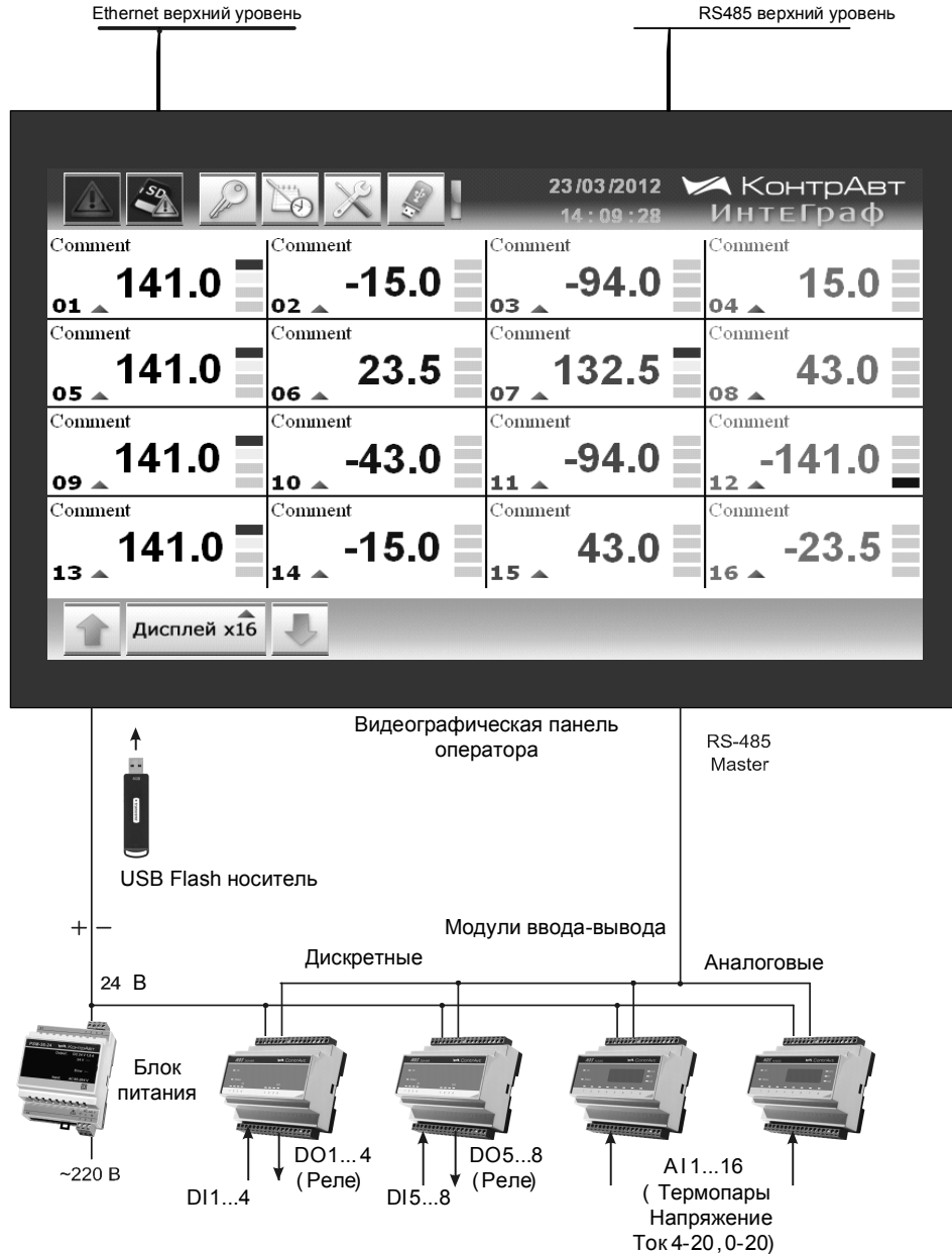
Рисунок 1 – Состав и структура Станции
