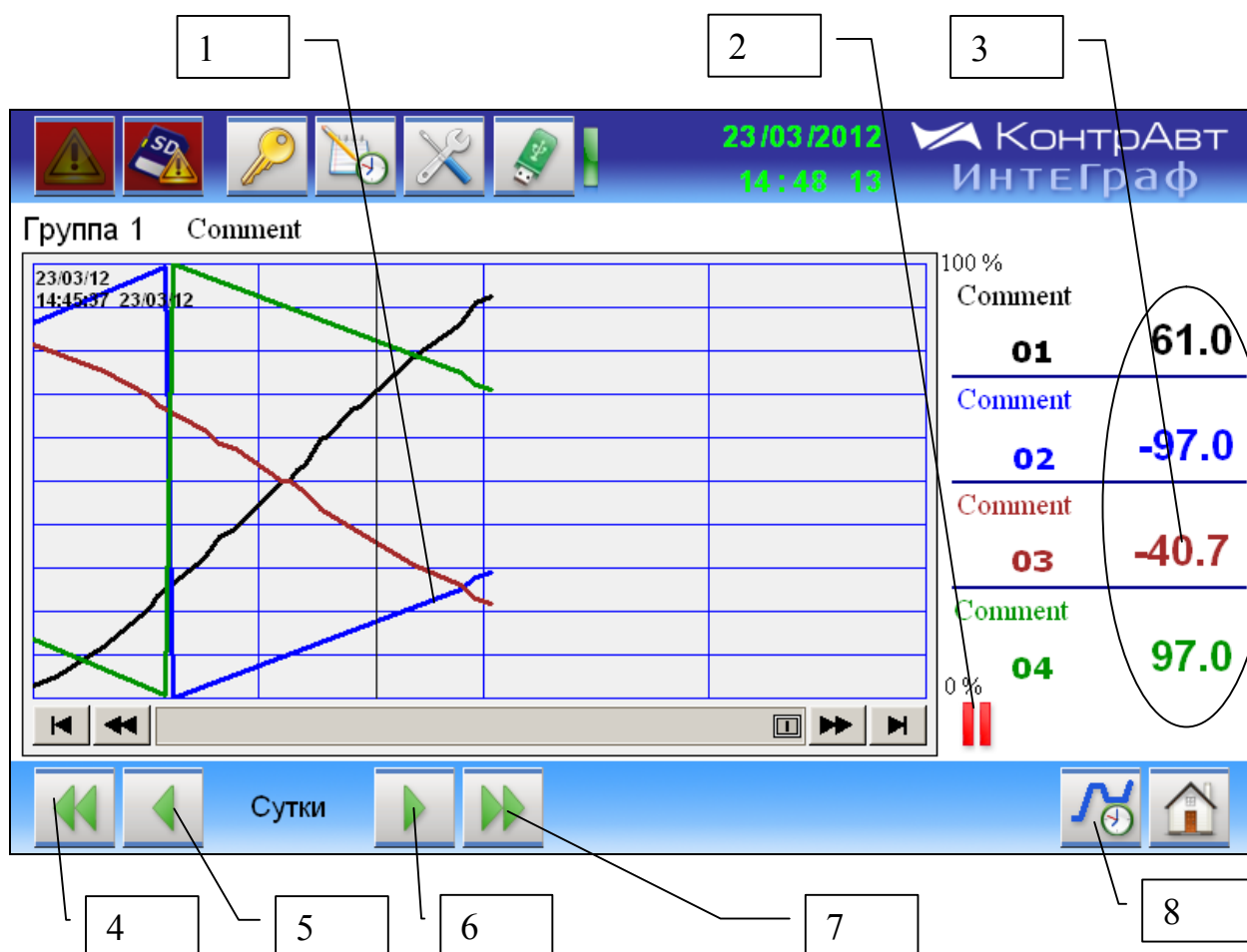
Рисунок 15 – Архивный Групповой тренд аналоговых сигналов
