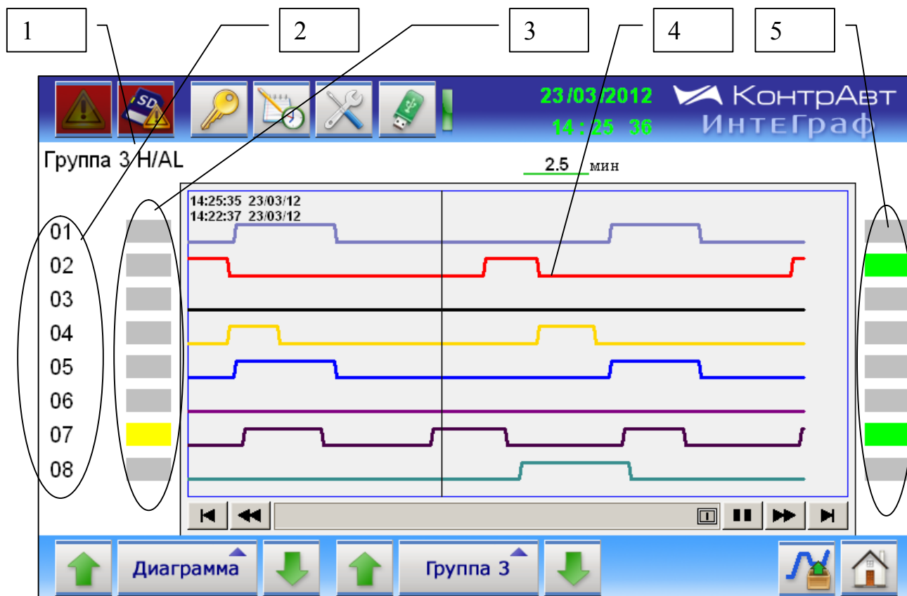
Рисунок 12 – Внешний вид экрана Группового тренда дискретных сигналов ( Диаграмма )
