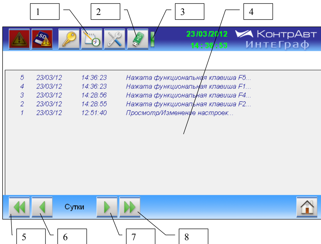
Рисунок 14 – Внешний вид экрана Архивного Журнала Событий .
