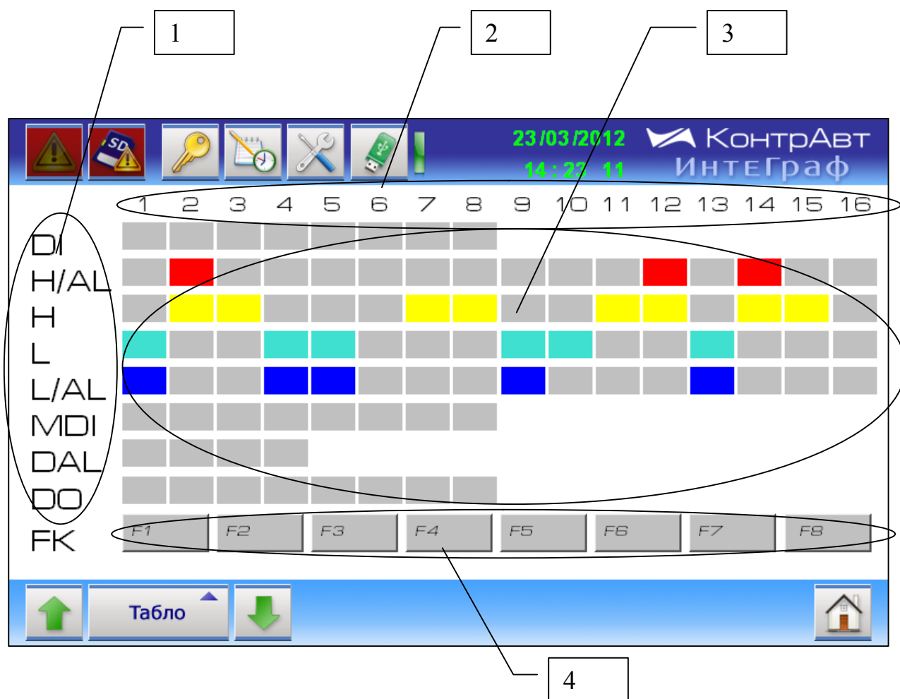
Рисунок 11 – Внешний вид экрана отображения дискретных сигналов ( Табло ).
