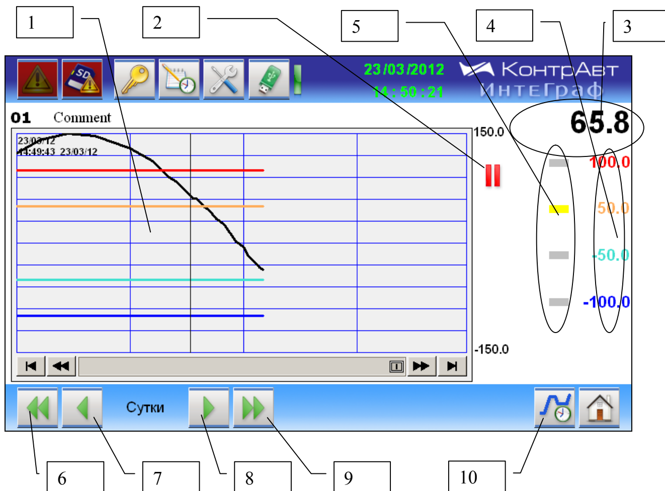
Рисунок 16 – Внешний вид экрана Архивный Единичный тренд аналогового сигнала
