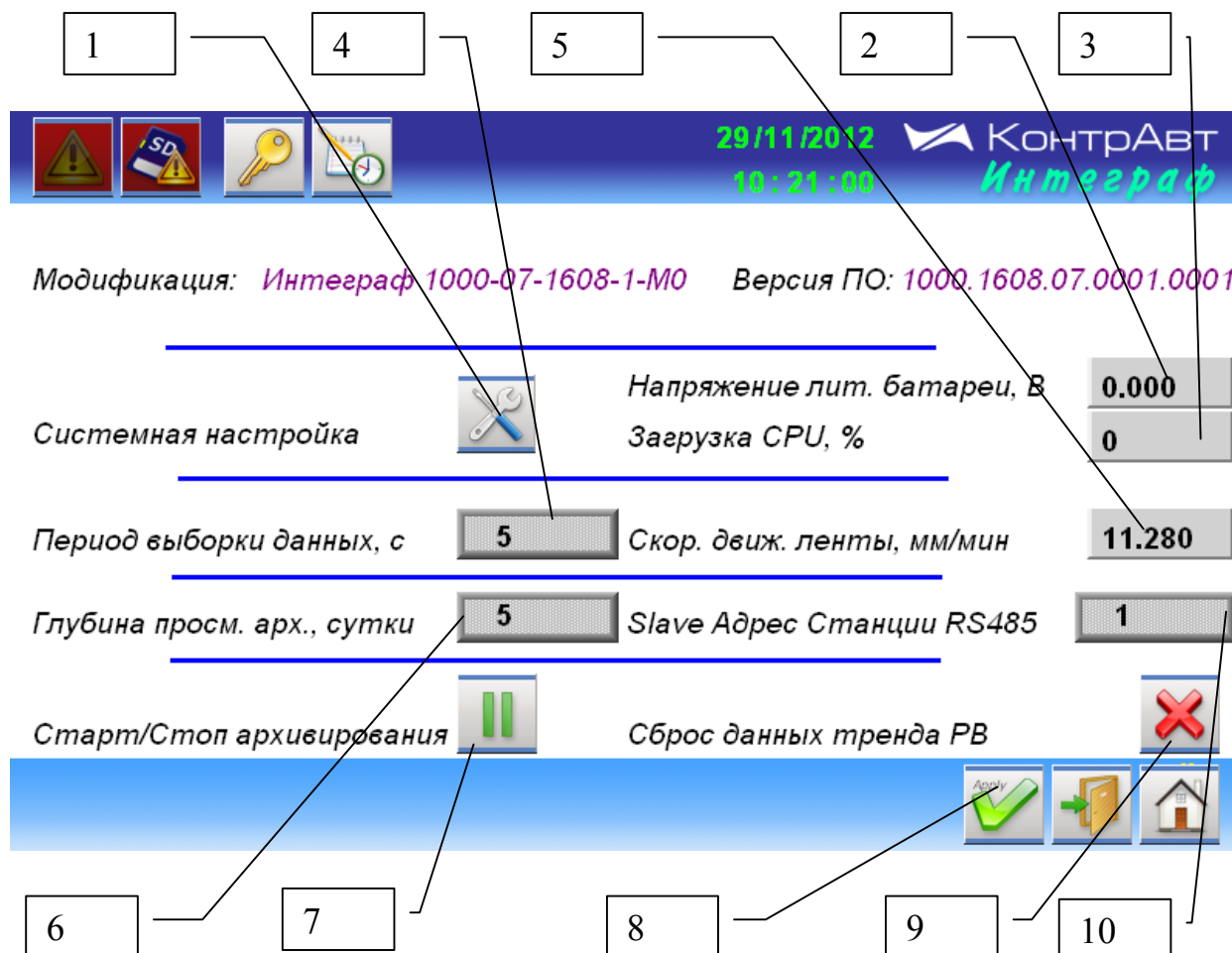
Рисунок 22 – Внешний вид экрана Настройка Общая
