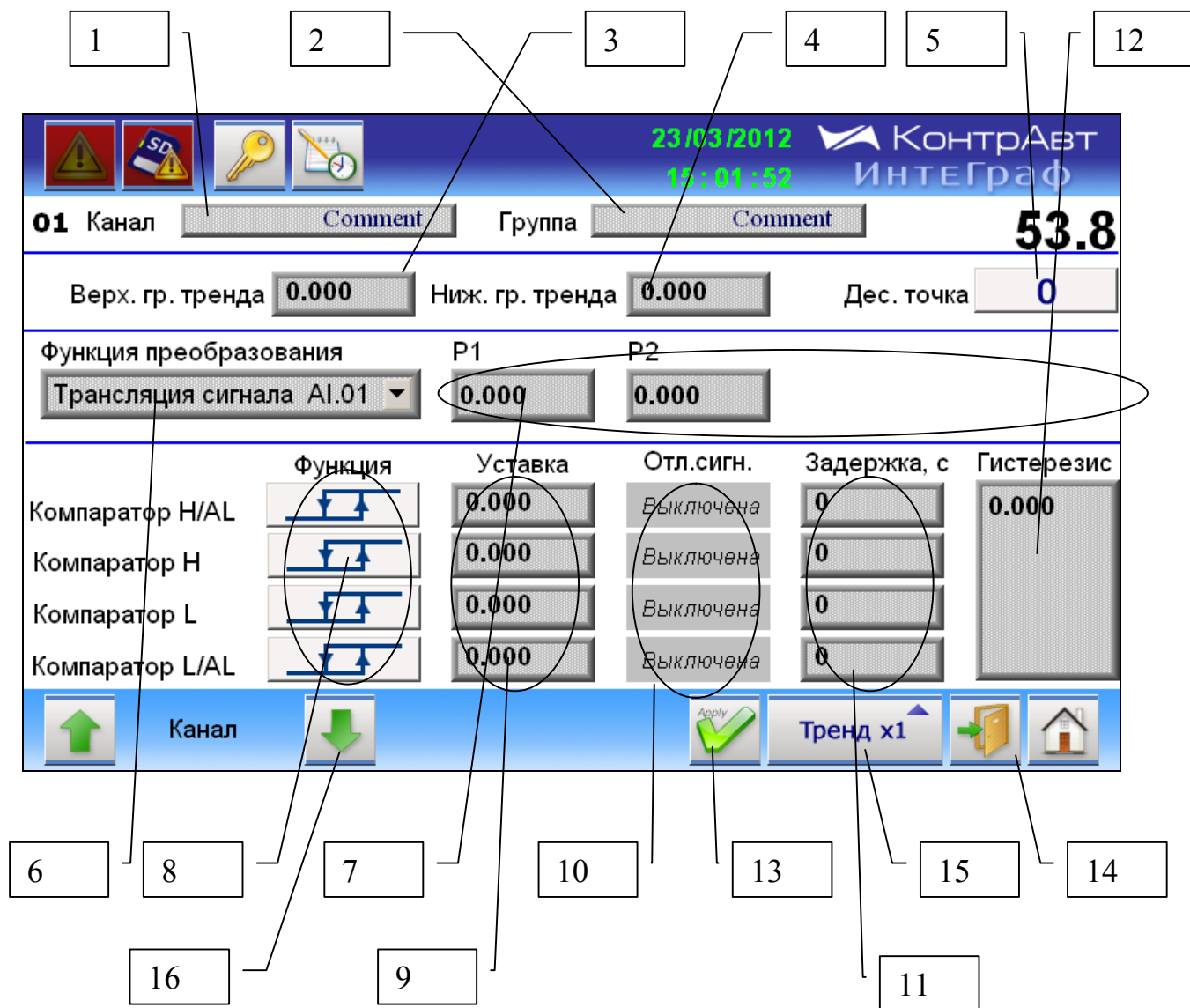
Рисунок 18 – Внешний вид экрана Настройка Аналогового измерительного канала
