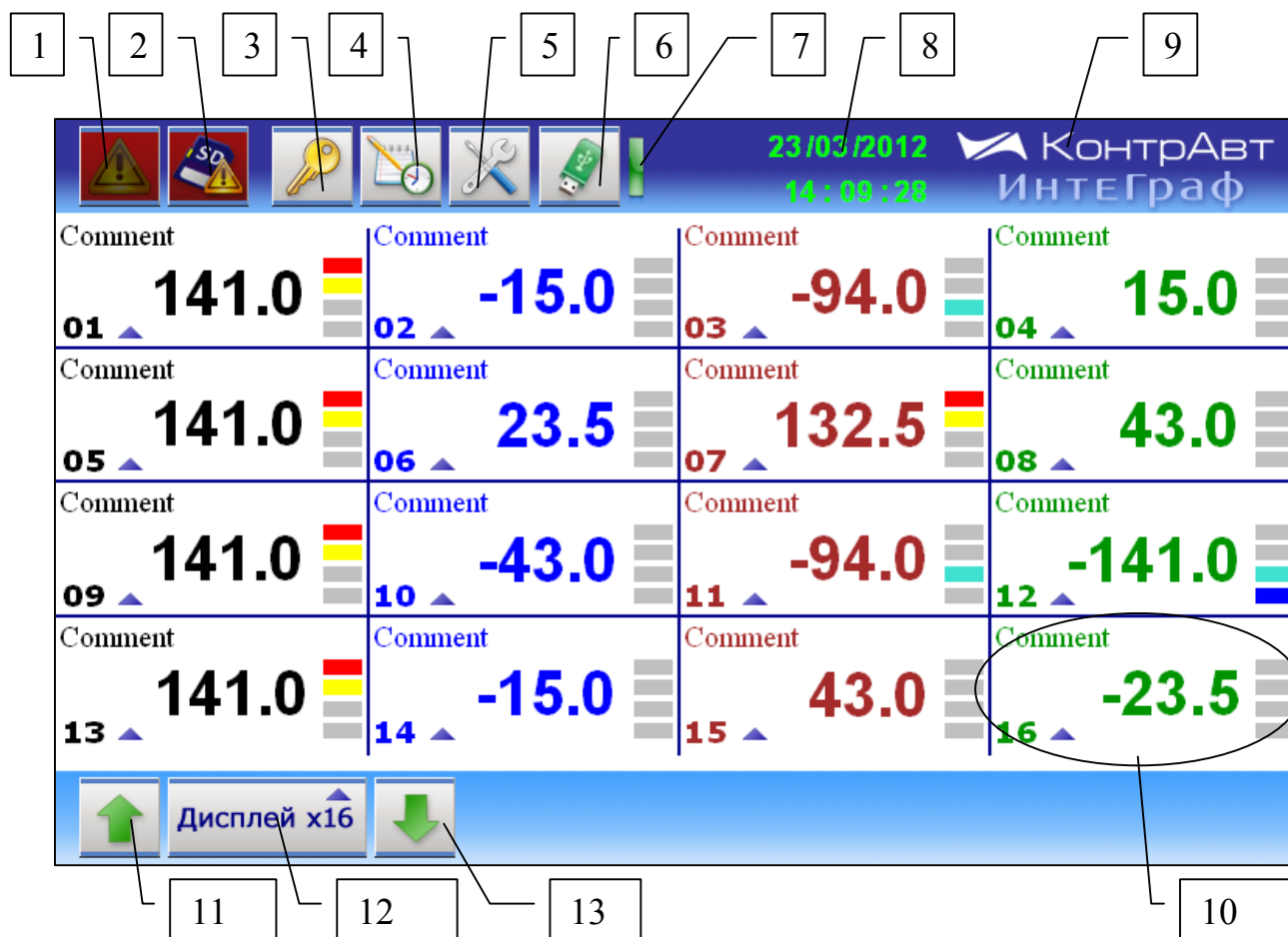
Рисунок 6 – Внешний вид основного экрана
