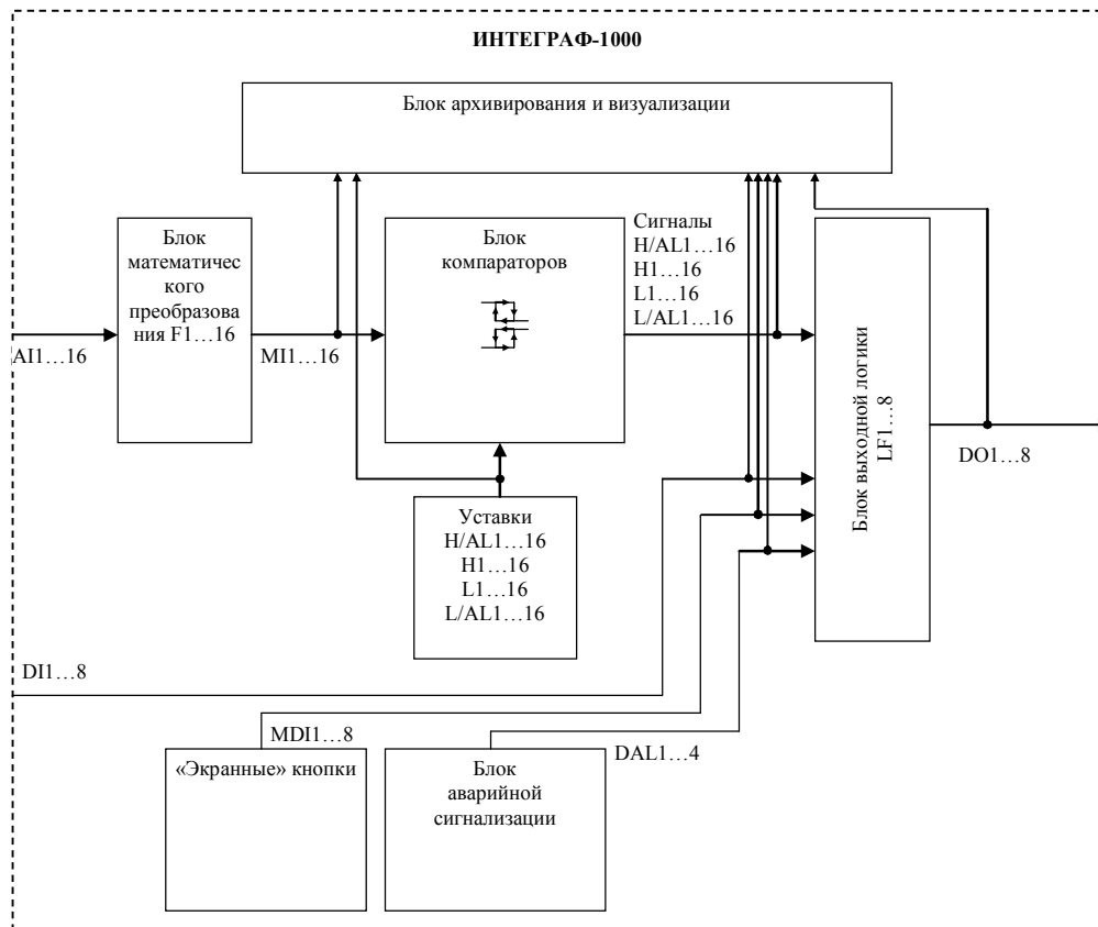
Рисунок 2 – Функциональная структура Станции
