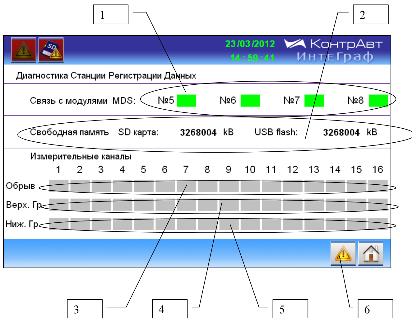
Рисунок 17 – Внешний вид экрана Диагностика
