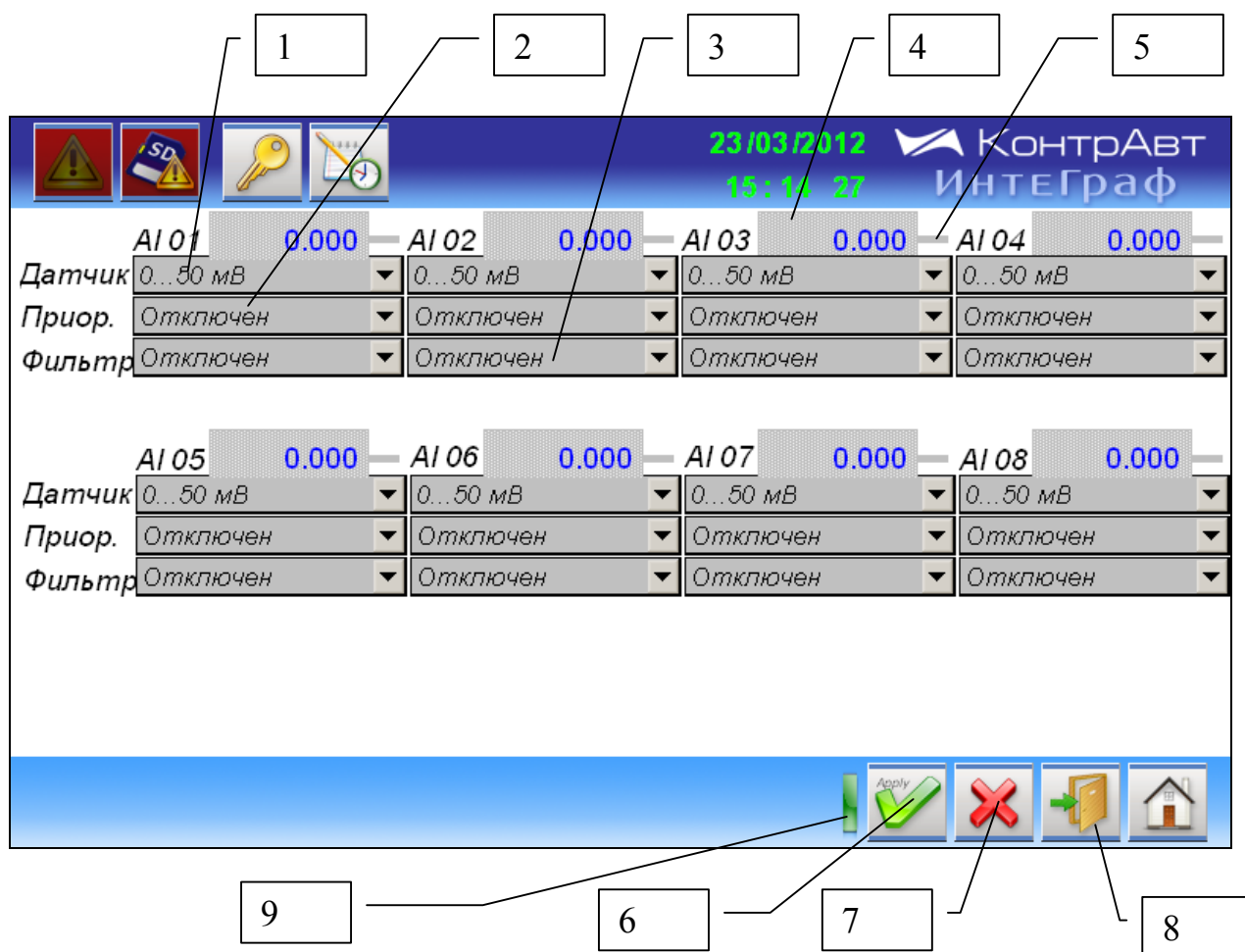
Рисунок 20 – Внешний вид экрана Настройка аналоговых входов модуля MDS AI-8TC
