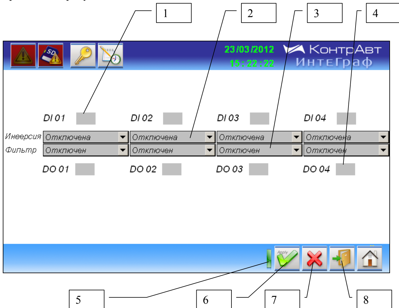
Рисунок 21 – Внешний вид экрана Настройка дискретных входов модуля MDS DIO-4/4R
