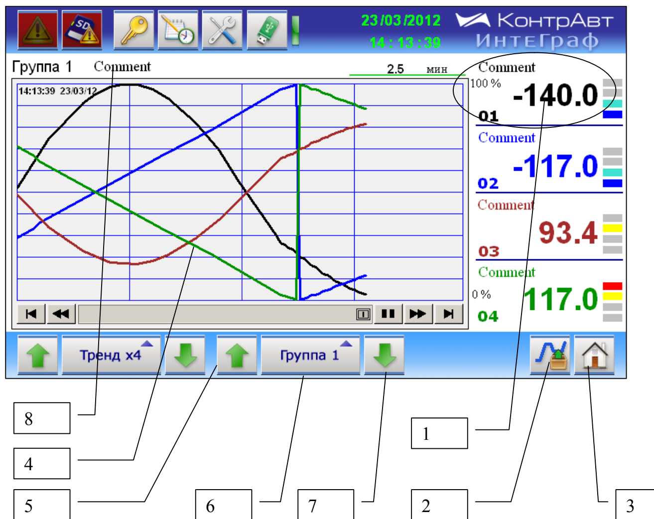
Рисунок 7 - Внешний вид экрана Группового тренда аналоговых измеренных сигналов ( Тренд x4 )
